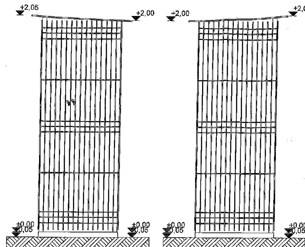
FATADA LATERALA DREAPTA scara 1:20
