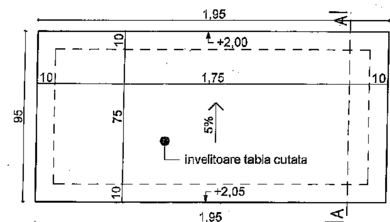
PLAN INVELITOARE scara 1:20
